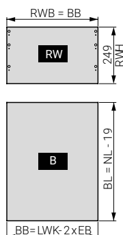
Einbaumaße Rückwand | Schnittmaße
