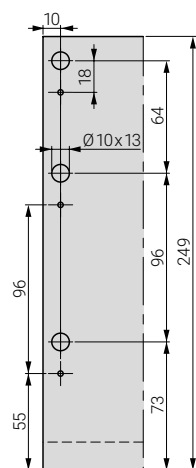
Einbaumaße Rückwand | Schnittmaße
