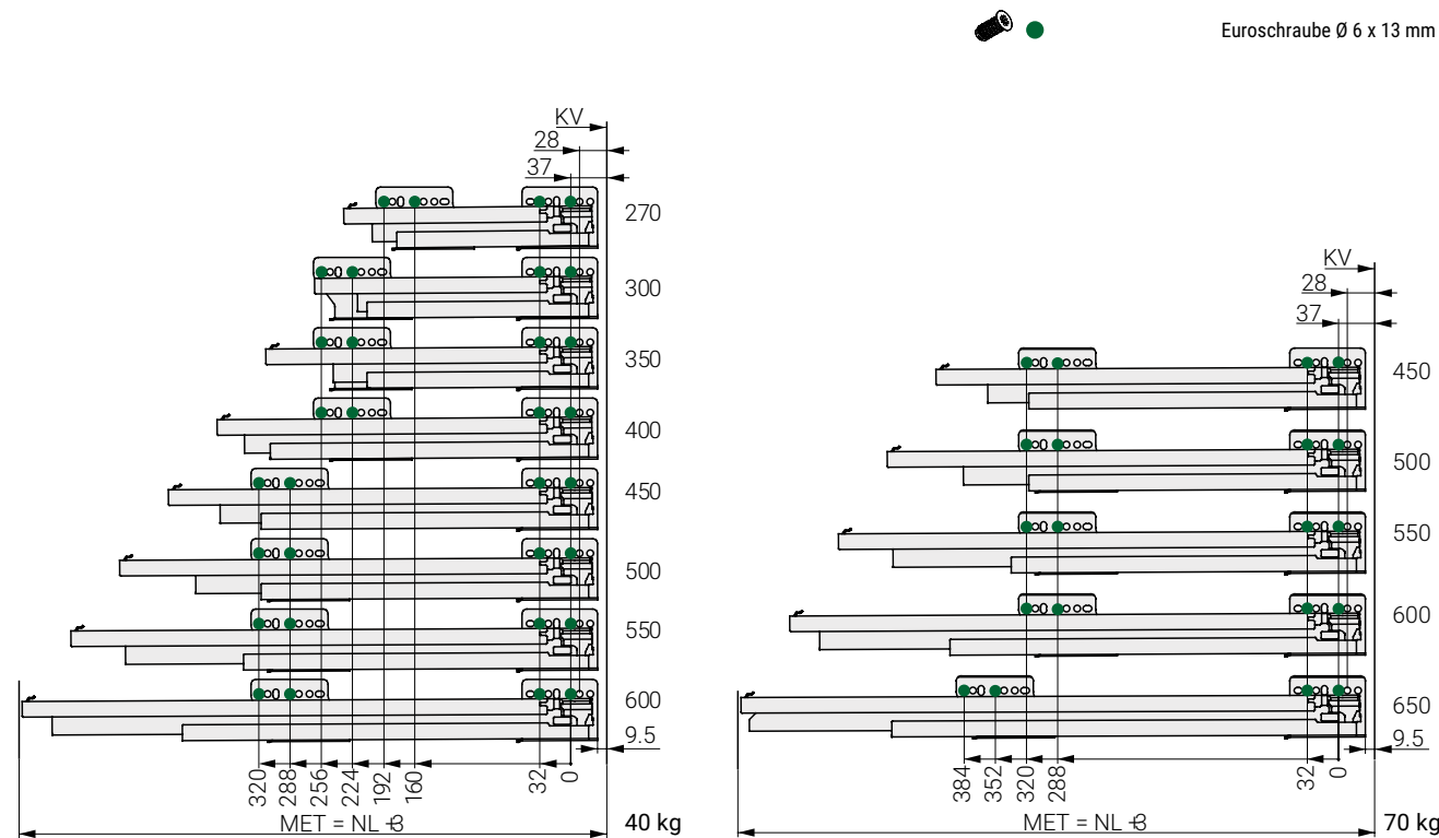
Befestigungsposition der Führungen auf die Schublade
