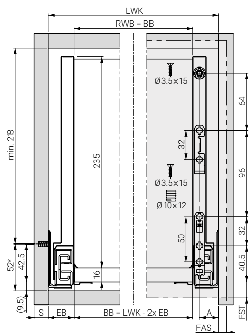
Einbaumaße der Schublade
